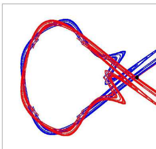
Figura 3. Enredo homoclínico
